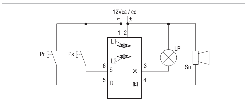
Šema povezivanja 441087C Connection Diagram 441087C
