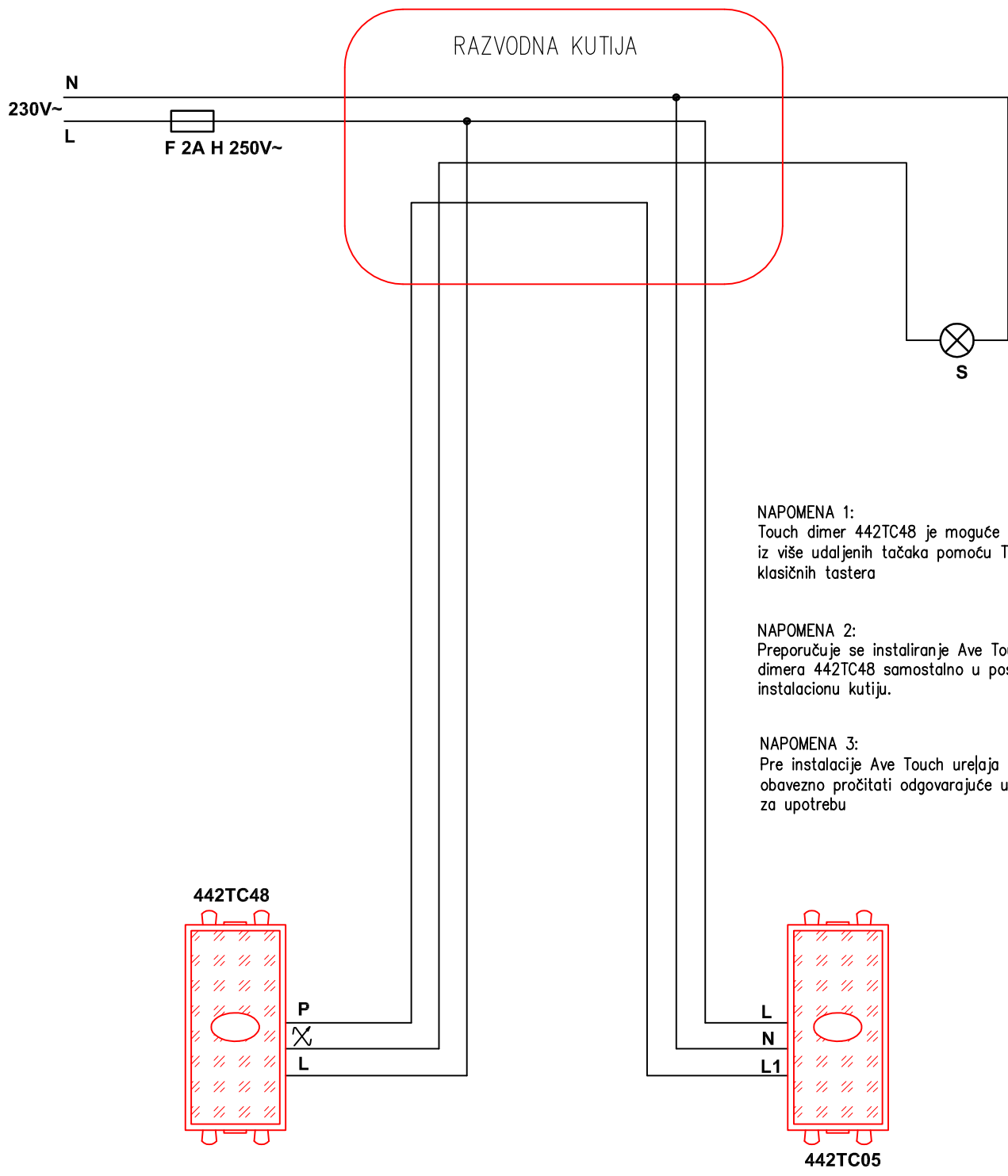
Kontrola Touch dimera 442TC48 pomoću Touch tastera 442TC05
