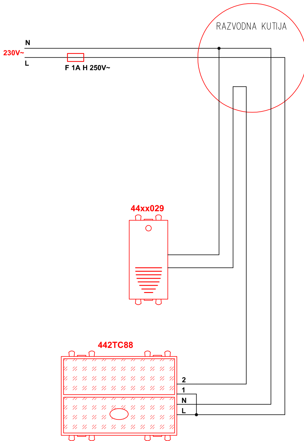
Kombinacija Ave Touch tastera za zvono 442TC88 i elektromehaničkog zvona 44x029 na 230Vac
