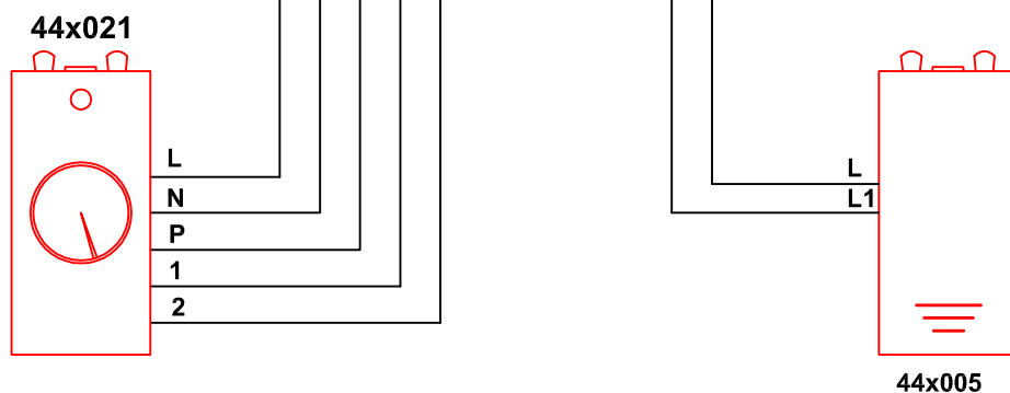
Kontrola elektronskog tajmere 44x021 pomoću tastera 44x005
