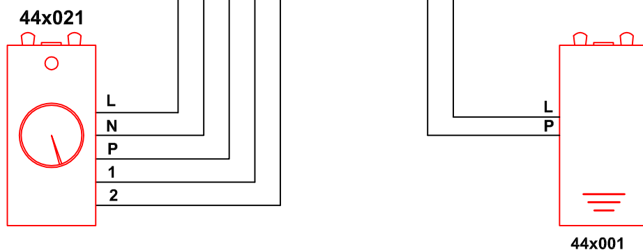
Kontrola elektronskog tajmere 44x021 pomoću običnog prekidača 44x001
